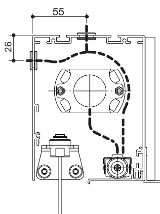
Box detail PM cable E115
