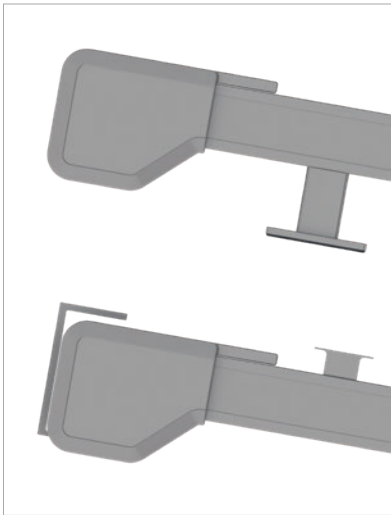
Kicsi dobozméret, 253×156 mm opcionális LED-del.
