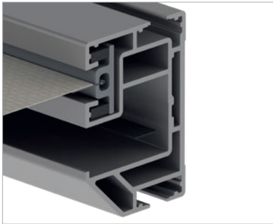
Hézagmentes vászonvezetés a protect kivételénél
