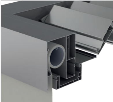
A palásttengely tökéletesen beépül a VENTUR szerkezetébe és bármikor utánszerelhető.
