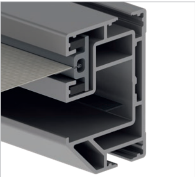
Opcionális résmentes vászonvezetés
