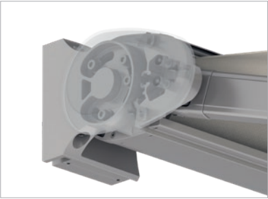
Nagy dőlésszög-tartomány a motoros meghajtású CLEO 5530 esetében falra szerelhető (6° – 65°) Mennyezetre szerelhető (5° – 80°)
