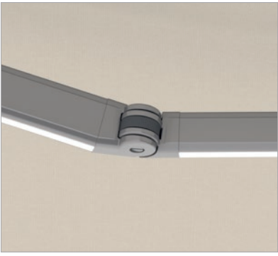
Csuklós kar eltakartan elhelyezkedő nagy szilárdságú húzószalaggal opcionálisan integrált LED világítással az AREIA 7040 esetében.
