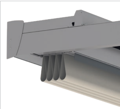
Díky speciálnímu vedení profilů pro textilií vyžaduje celý balík textilie o 20 procent méně místa než běžná zařízení.
