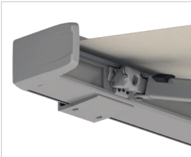
Sklopné ložisko ramene s pojistkou proti zdvihnutí při poryvu větru umožňuje spolehlivé uzavírání a zabraňuje nadzvednutí při nárazovém větru.
