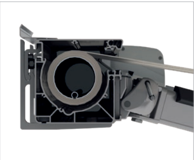
Jednodílný profil kazety pro textilií zabraňuje torzi kazetové markýzy a umožňuje optimální napojení na stěnu.
