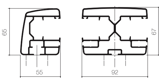
tenda plus B (Schräg-/Senkrechtanlage)
