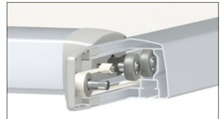
Führungsschiene und Teil des Spannsystems
