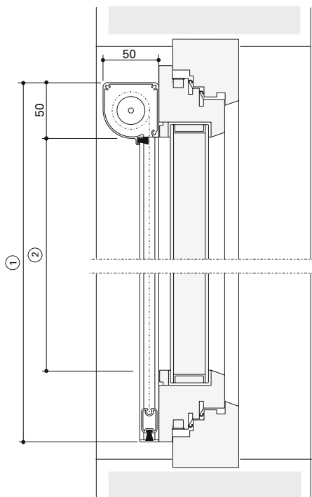
Montage von vorne auf den Fensterflügel
