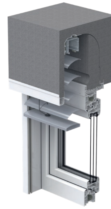
TOP FOAM store S integriranim otvorom za prihvat vanjskih raffstore žaluzina
