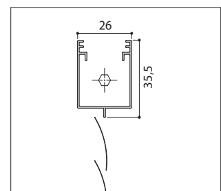
Oberschiene mit Steg zur Reduktion des Lichtspaltes zur obersten Lamelle
