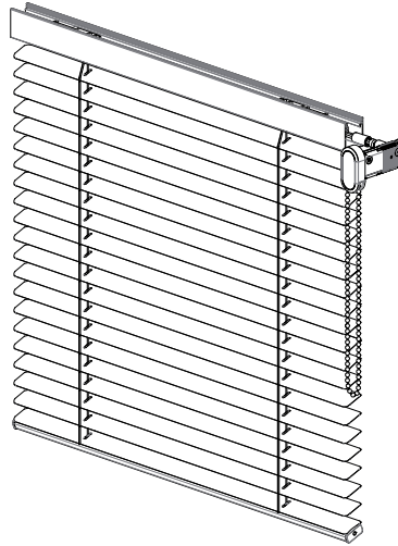
JVF 25 KZD Verbundfensterjalousie mit Kettenzugantrieb**
